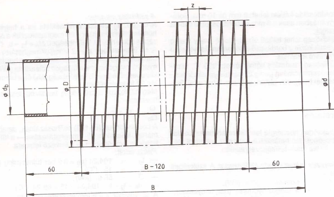
1. ábra Az ASB típusjelű bordáscső körvonalrajza
