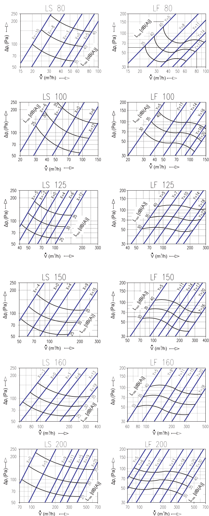
2.31-2 ábra LS / LF Légszelepek kiválasztása
