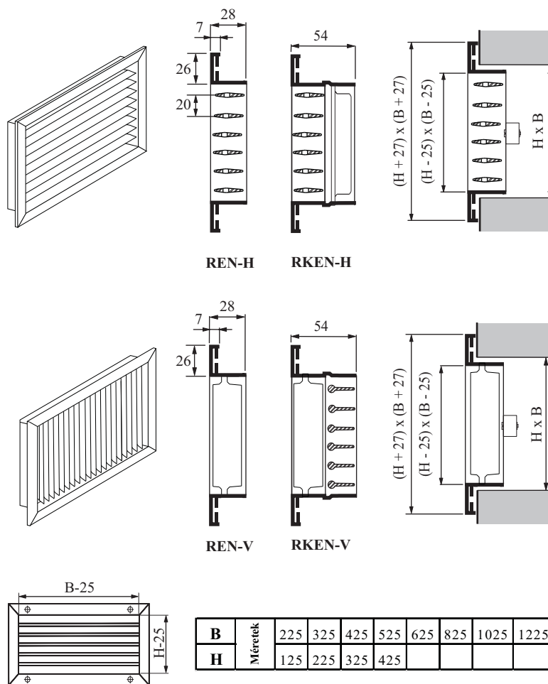
2.11-1 ábra REN / RKEN rácsok fő méretei
