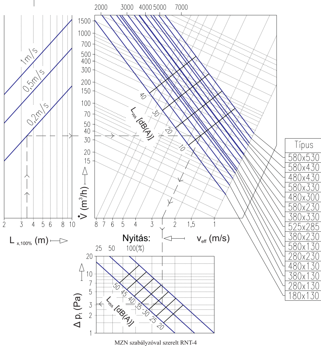
2.21-4. diagram RNT-4 négyszög anemosztát kiválasztása
