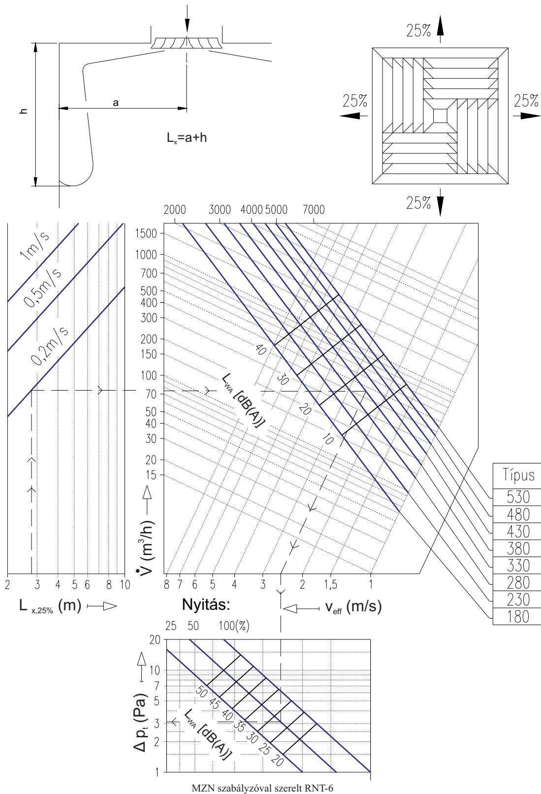
2.21-6. diagram RNT-6 négyszög anemosztát kiválasztása
