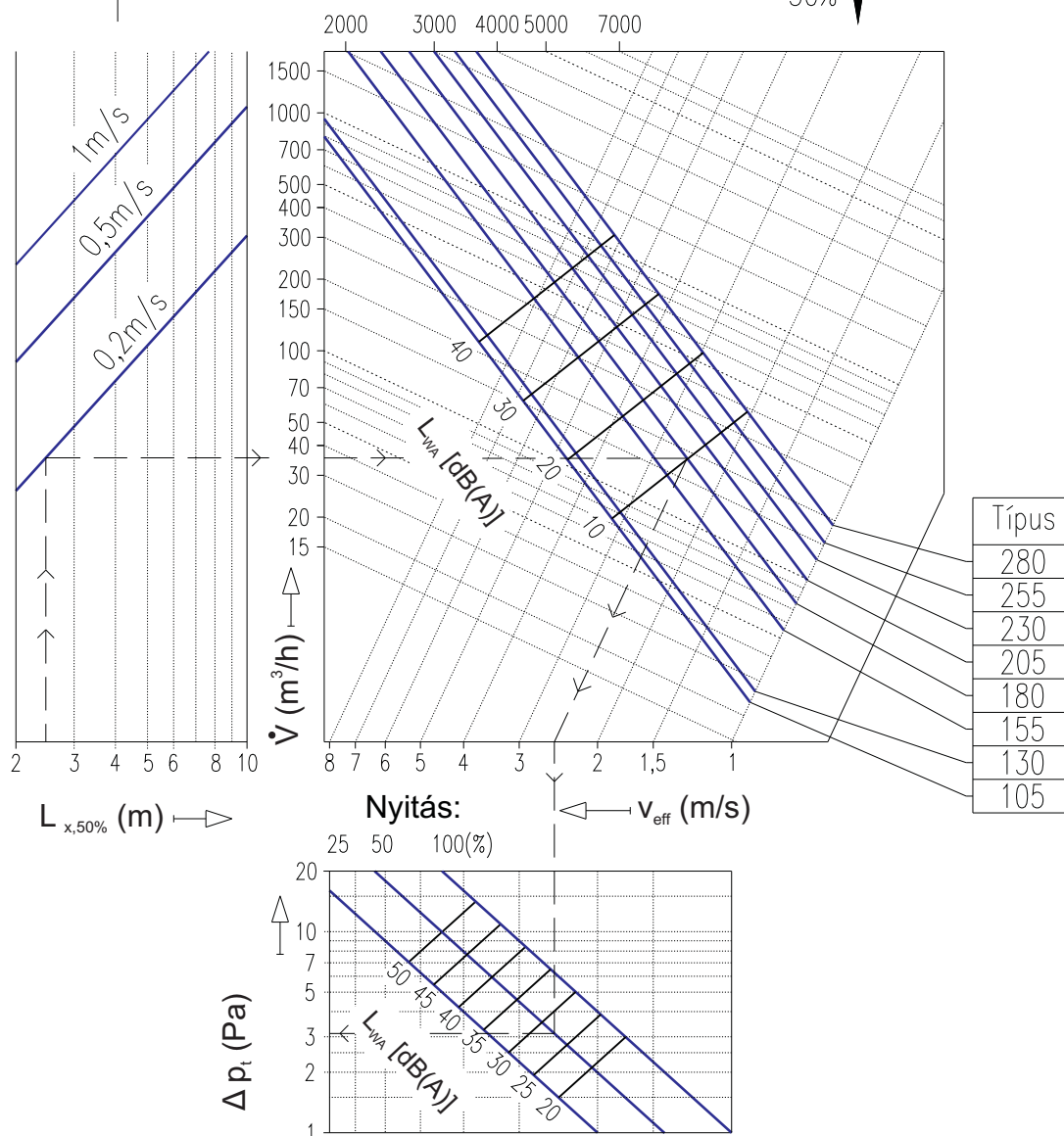
2.21-3. diagram RNT-3 négyszög anemosztát kiválasztása
