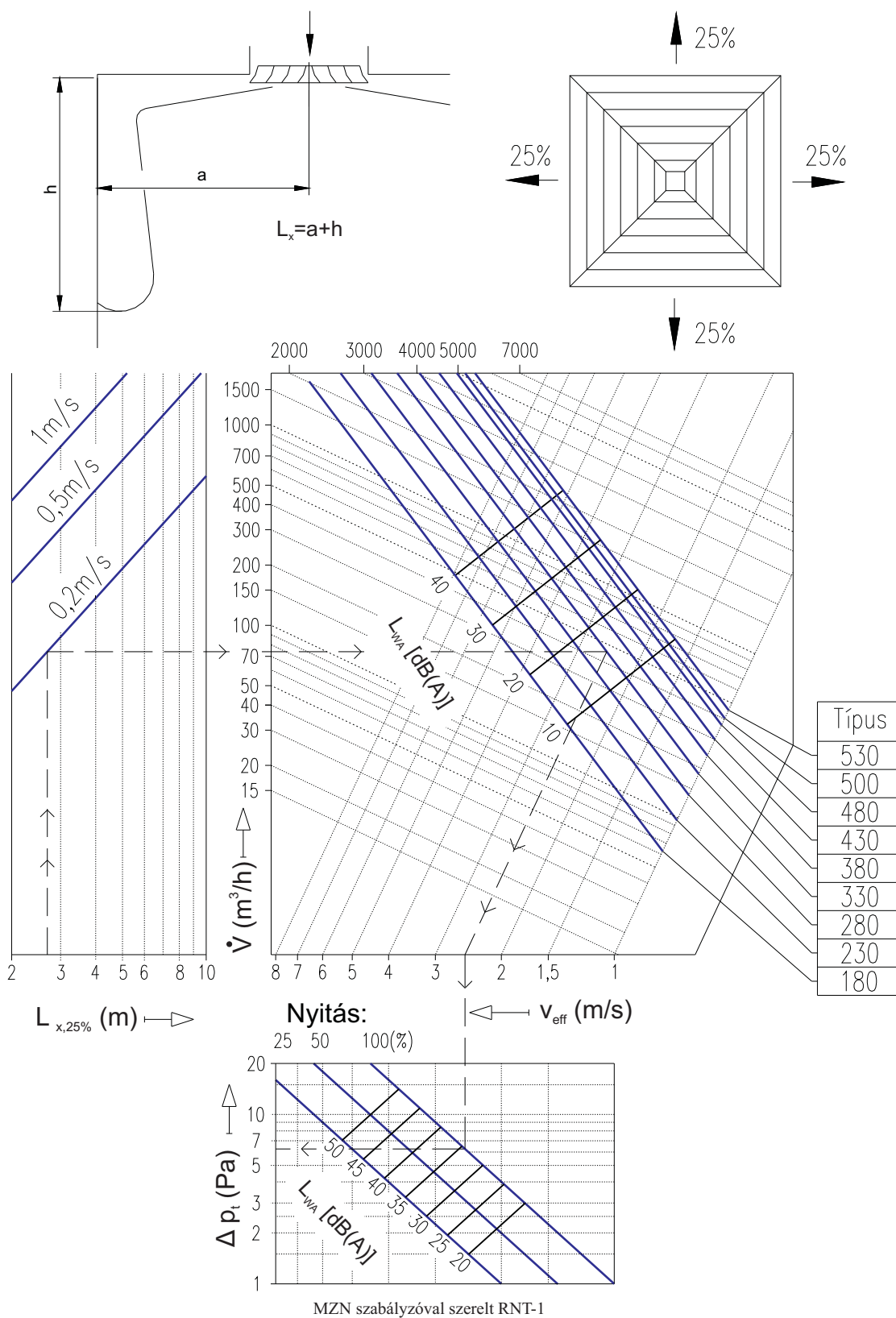
2.21-1. diagram RNT-1 négyszög anemosztát kiválasztása
