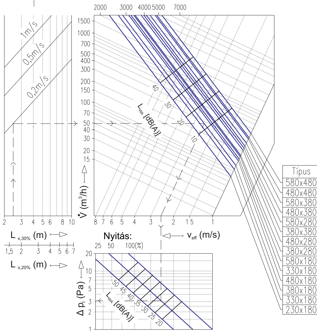
2.21-7. diagram RNT-7 négyszög anemosztát kiválasztása
