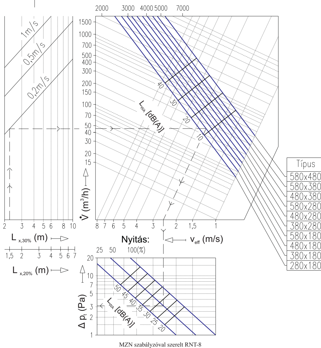
2.21-8. diagram RNT-8 négyszög anemosztát kiválasztása
