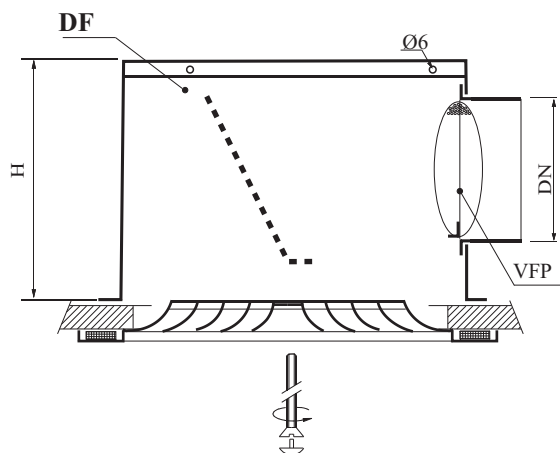
DF dobozokkal szerelt RNT anemosztát
