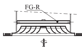
Felszerelés csövégre FG-R rúddal
