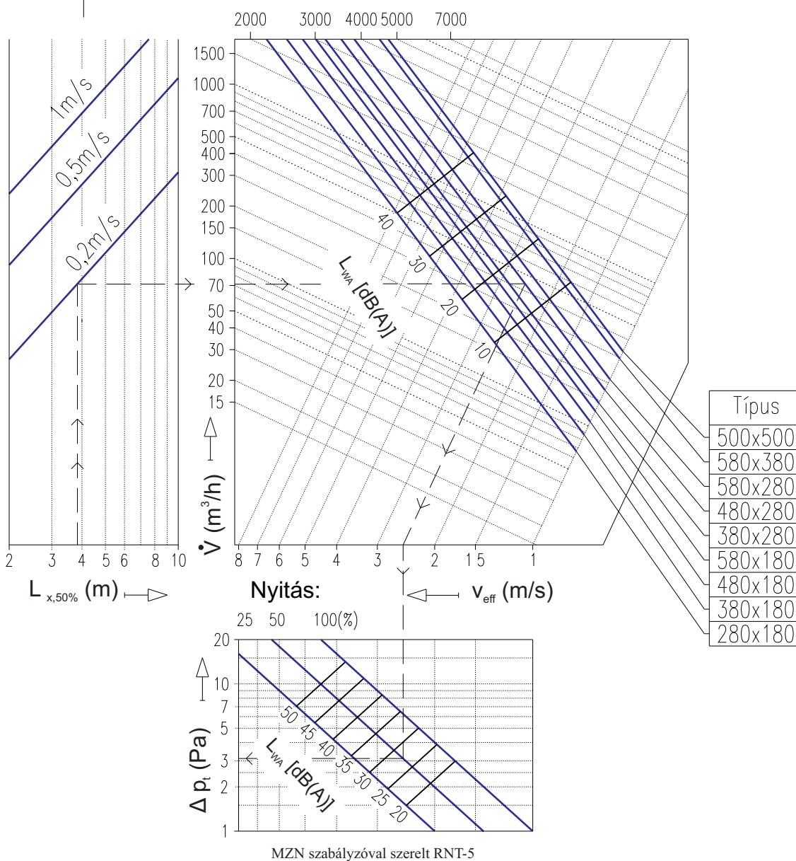
2.21-5. diagram RNT-5 négyszög anemosztát kiválasztása
