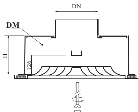
DM dobozokkal szerelt RNT anemosztát
