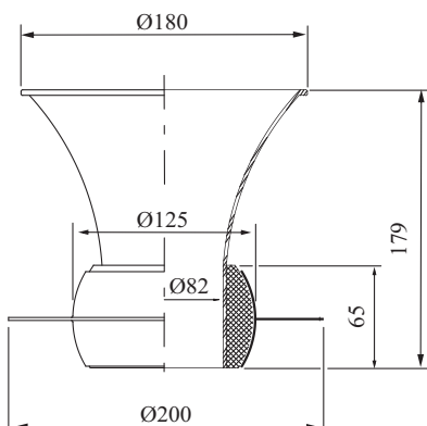
2.32-3 ábra SF-200 sugárfúvókák fő méretei és kiválasztása
