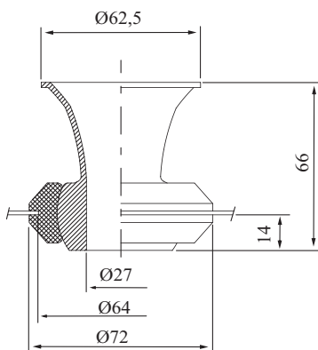
2.32-2 ábra SF-20 sugárfúvókák fő méretei és kiválasztása
