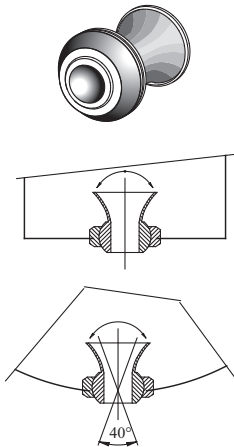
2.32-2 ábra SF-20 sugárfúvókák fő méretei és kiválasztása
