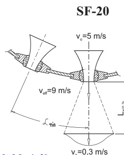
2.32-4 ábra SF-20 sugárfúvókák SPIKO kör légszatórnára szerelve
