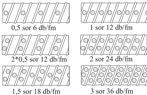
2.32-4 ábra SF-20 sugárfúvókák SPIKO kör légszatórnára szerelve
